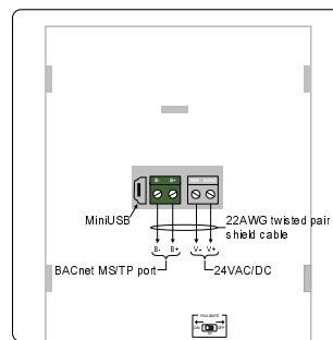
Fig. 2 DST35U Port
