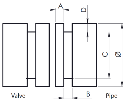
PS89 尺寸
