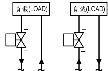
圖五 二通閥配置圖
