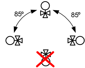
圖二 安裝角度示意圖
