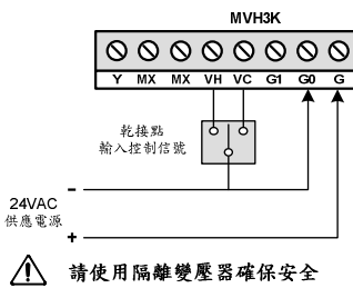
圖三 二位置式或浮動式控制接線圖
