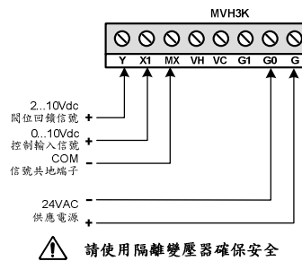
圖四 比例式控制接線圖
