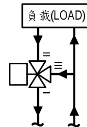
圖五 三通閥配置圖
