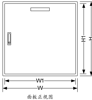
单门右开式(CP-S)
