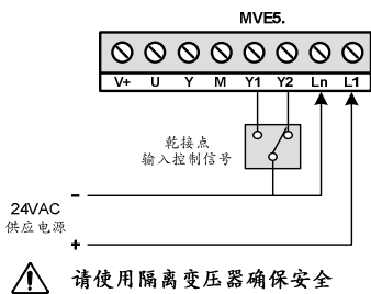
图三 二位置或浮动式控制接线图
