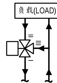
图五 三通阀配置图
