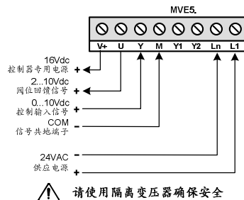
图四 比例式控制接线图
